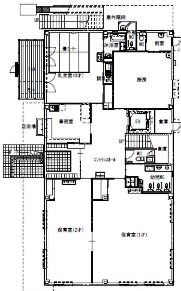
1階平面図 S = 1 : 250
