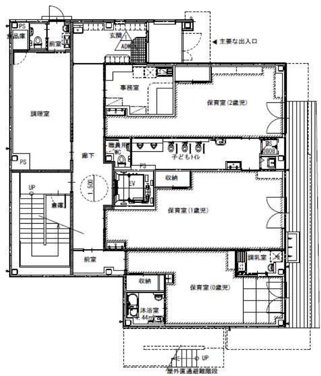
平面図
