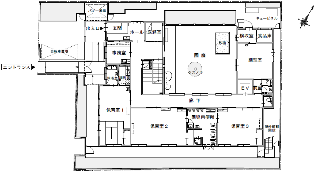
1 階 平 面 図
